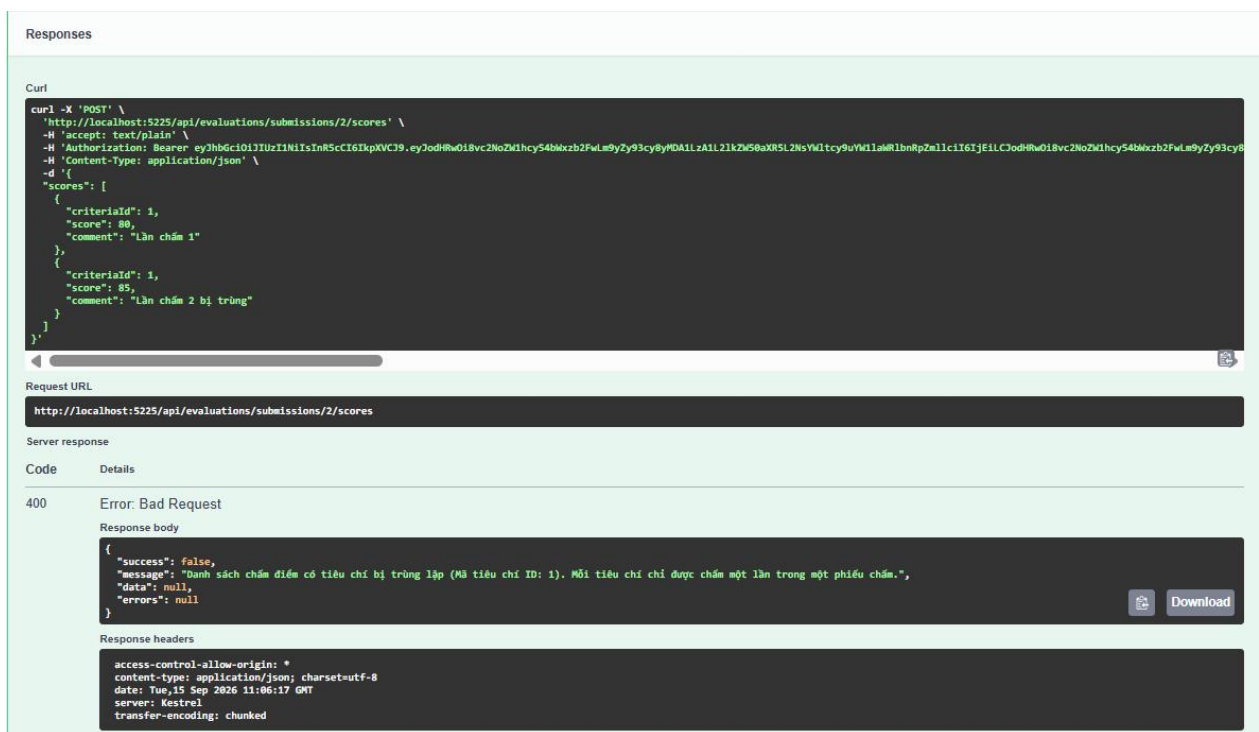
Hình 6. Thử gửi Trùng lặp Tiêu chí trong cùng 1 Phiếu chấm (response)
