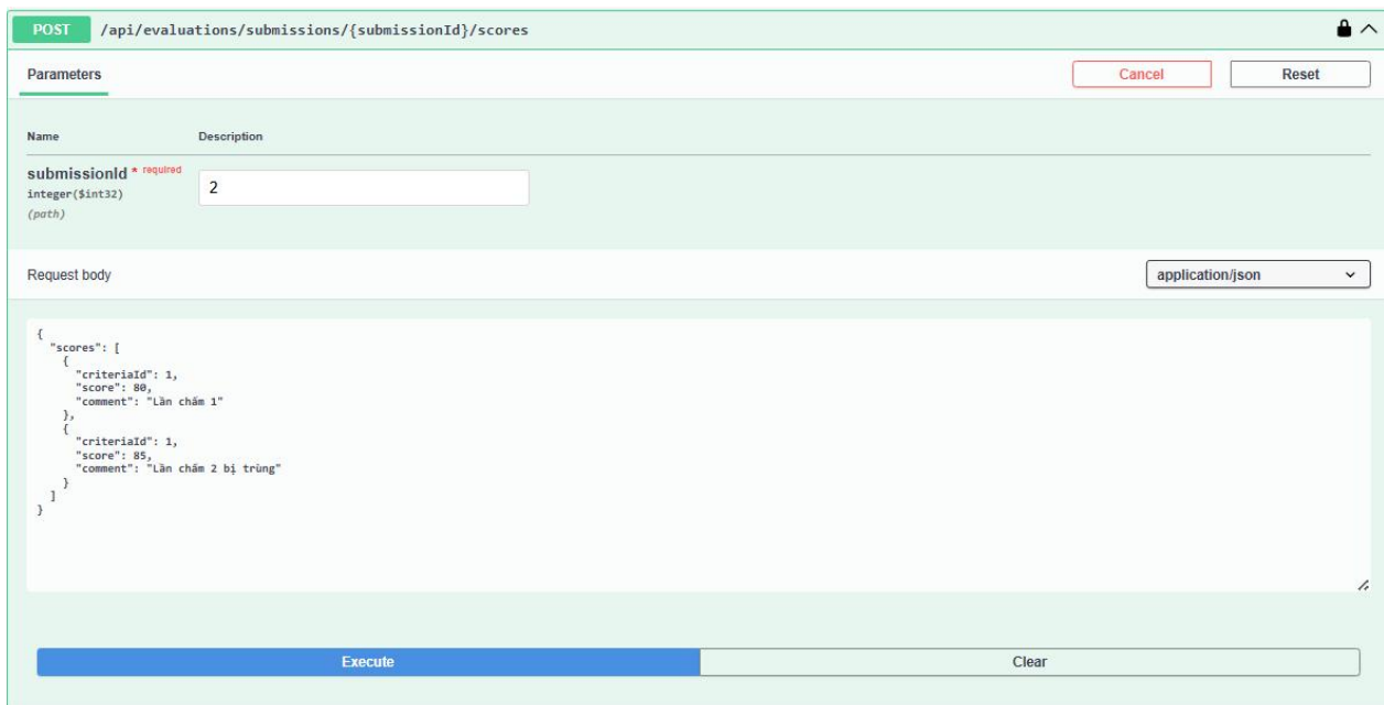
Hình 5. Thử gửi Trùng lặp Tiêu chí trong cùng 1 Phiếu chấm (request)
