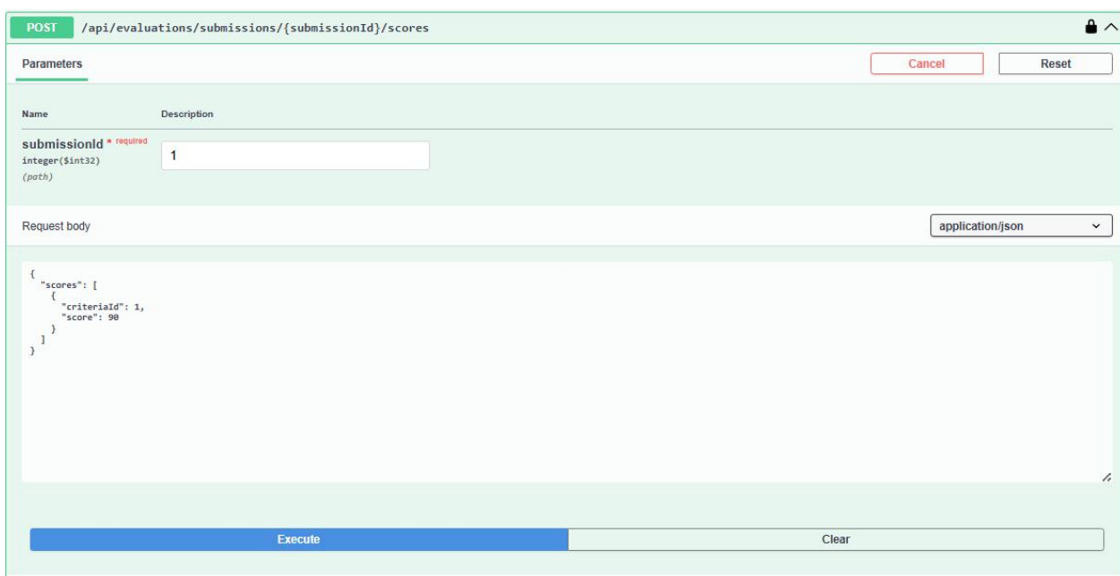
Hình 11. Chặn Sửa điểm Hồ sơ đã được duyệt Trúng thầu (request)
