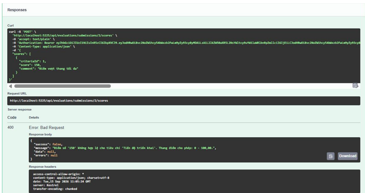
Hình 4. Thử chấm Điểm vượt Thang điểm tối đa (response)
