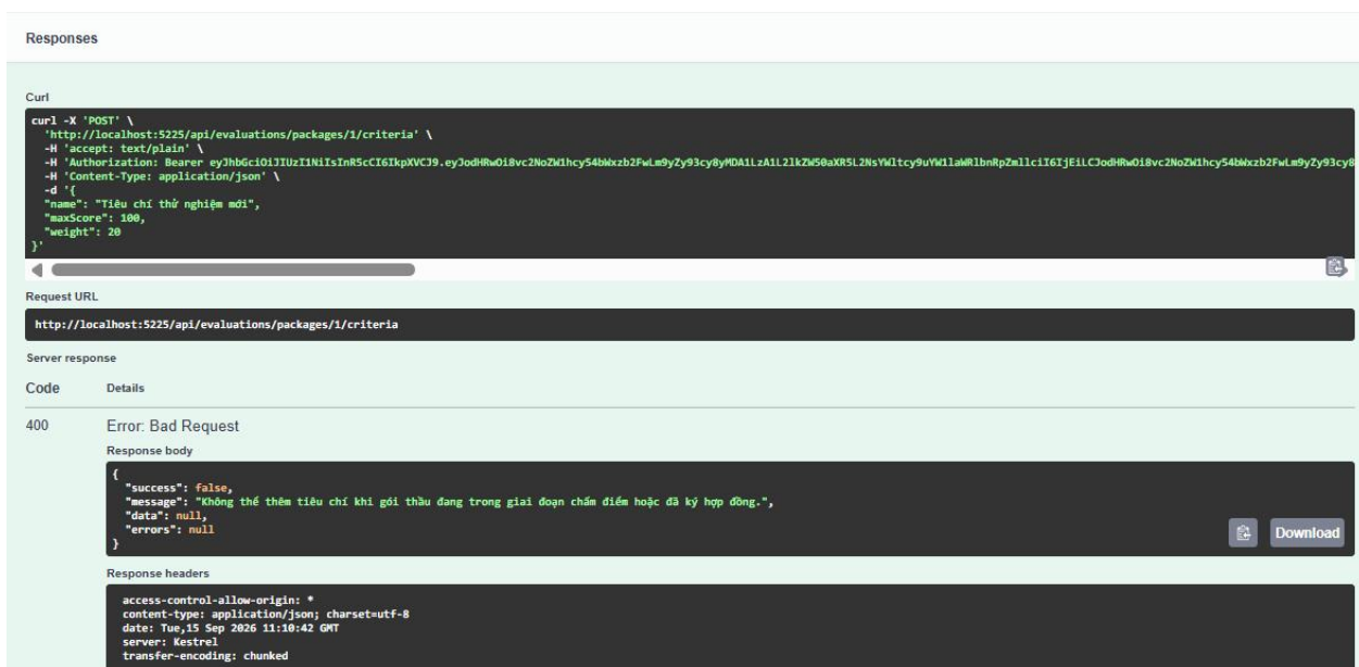
Hình 10. Chặn Thêm tiêu chí khi gói thầu đã chuyển sang giai đoạn Chấm điểm (response)
