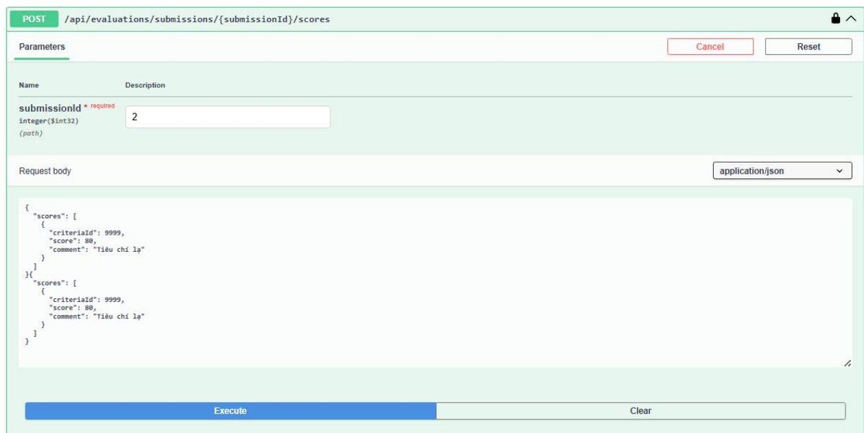
Hình 7. Thử chấm Tiêu chí không thuộc gói thầu (request)
